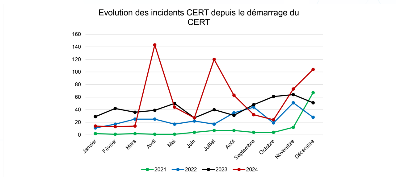
Graphique 6 : Évolution des incidents CERT par mois
